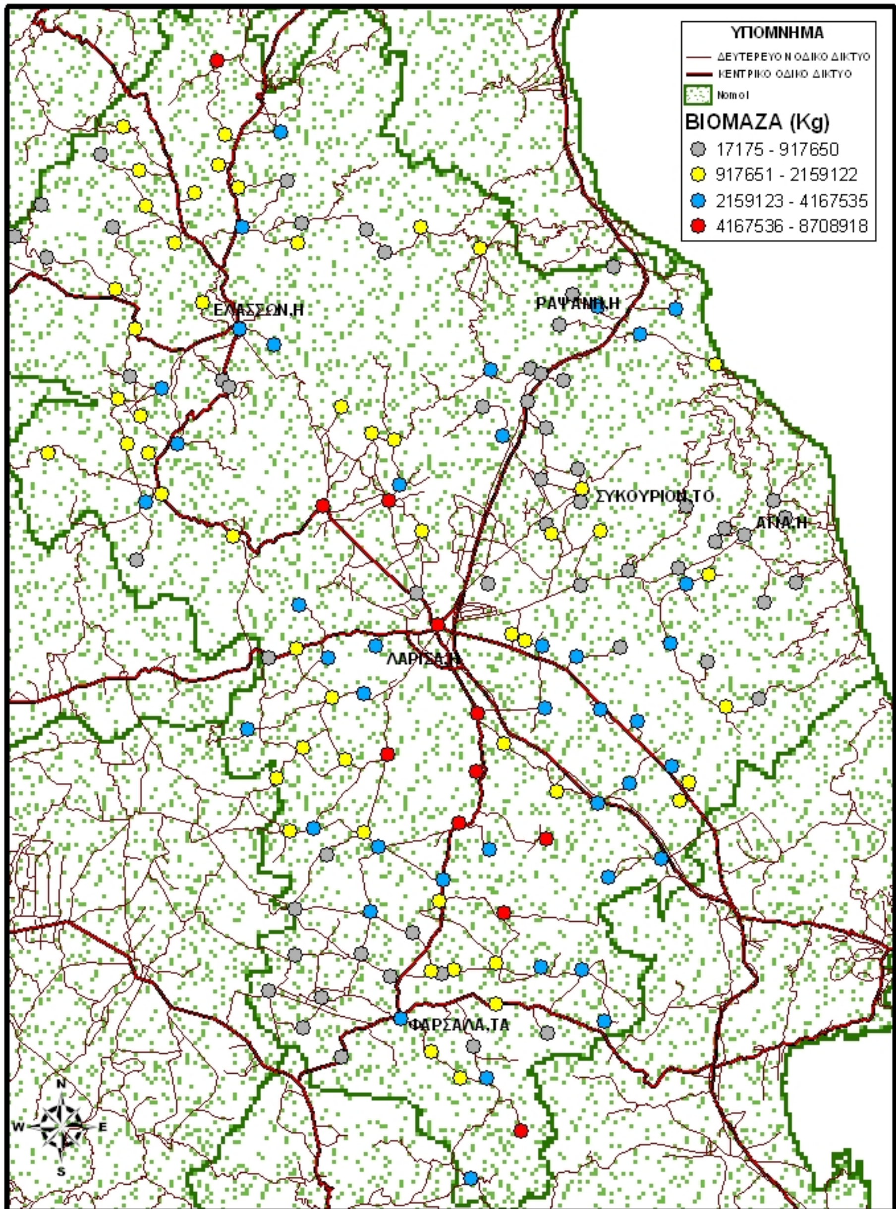
ΧΑΡΤΗΣ 3: ΠΑΡΑΓΩΓΗ ΒΙΟΜΑΖΑΣ ΑΠΟ ΥΠΟΛΕΙΜΜΑΤΑ ΣΠΗΡΩΝ
